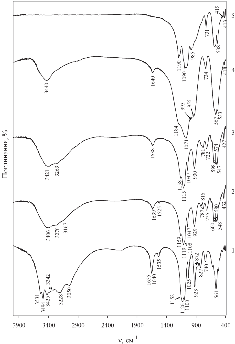
Рис. 2. ІЧ-спектри продуктів термолізу \text{Co}_{0.16}\text{Zn}_{0.39}\text{P}_2\text{O}_7 \cdot 6\text{H}_2\text{O} , одержаних за 358 (1), 463–513 (2), 558 (3), 698 (4), 843–1273 К (5)
