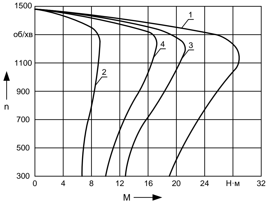
Рис. Механічні характеристики трифазного асинхронного електродвигуна:
