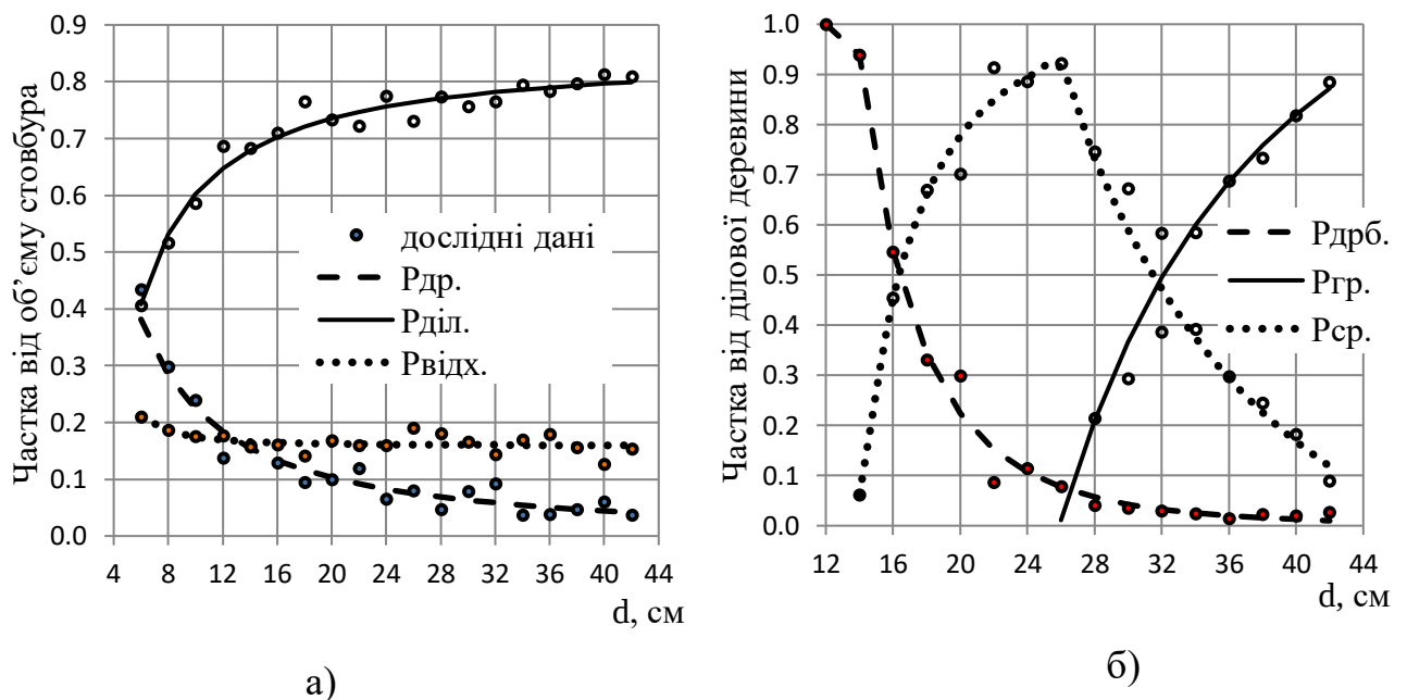
Рис. 2. Математичні моделі розмірно-якісної структури (а - за категоріями деревини, б – ділової деревини за категоріями крупності)
